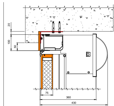
DETTAGLIO TELAILO PARZIALMENTE IN LUCE SEZIONE VERTICALE IN BETWEEN PARTIAL INSTALLATION VERTICAL SECTION
