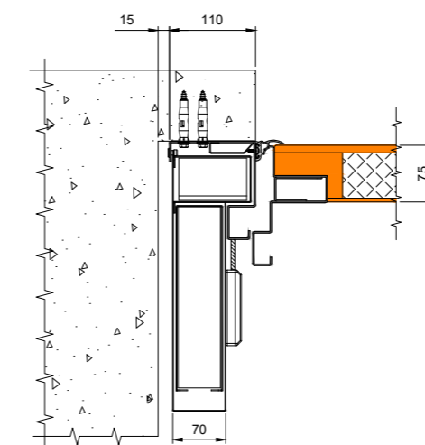
DETTAGLIO TELAILO OLTRE LUCE IN BATTUTA SEZIONE ORIZZONTALE WALL BEHIND INSTALLATION HORIZONTAL SECTION
