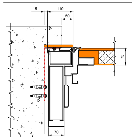
DETTAGLIO TELAILO PARZIALMENTE IN LUCE SEZIONE ORIZZONTALE IN BETWEEN PARTIAL INSTALLATION HORIZONTAL SECTION
